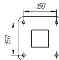
ПЛАН ОБОРУДОВАНИЯ В ОСЯХ
