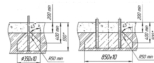
УСТАНОВКА СТОЕК ОБОРУДОВАНИЯ
