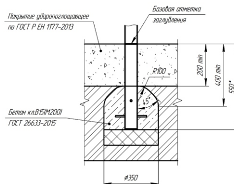
УСТАНОВКА ОБОРУДОВАНИЯ
