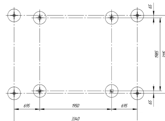
ПЛАН ОБОРУДОВАНИЯ В ОСЯХ
