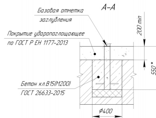
УСТАНОВКА СТОЕК ПРИ БЕТОНИРОВАНИИ
