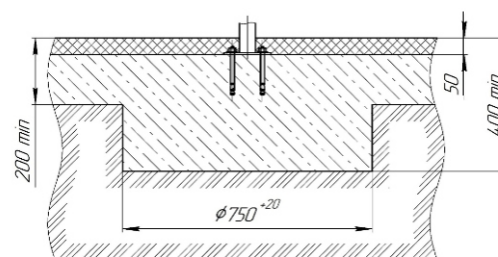
УСТАНОВКА СТОЕК ОБОРУДОВАНИЯ
