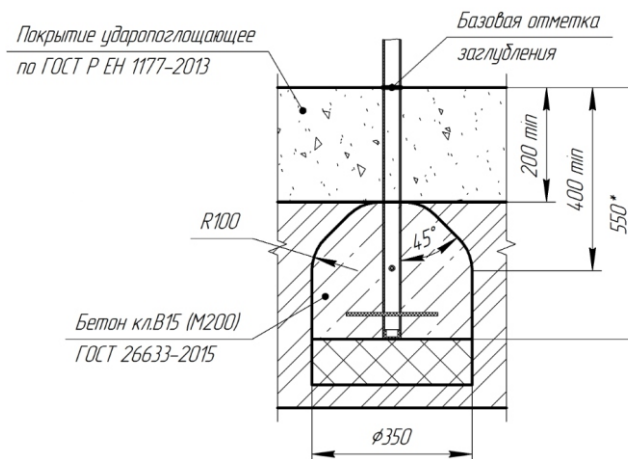
УСТАНОВКА СТОЕК ОБОРУДОВАНИЯ
