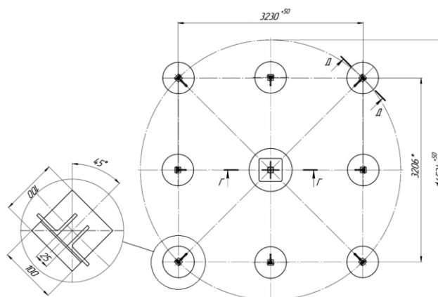
ПЛАН ОБОРУДОВАНИЯ В ОСЯХ
