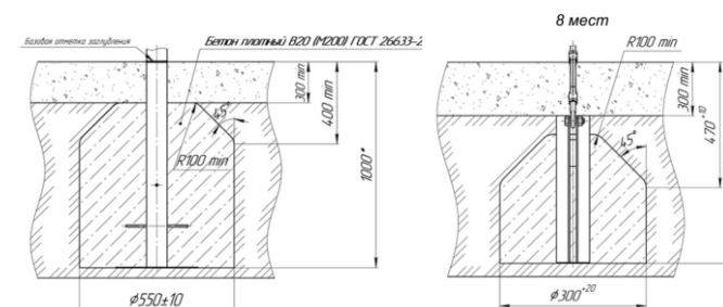
УСТАНОВКА СТОЕК ПРИ БЕТОНИРОВАНИИ
