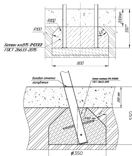
УСТАНОВКА СТОЕК ОБОРУДОВАНИЯ
