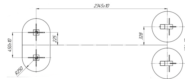
ПЛАН ОБОРУДОВАНИЯ В ОСЯХ
