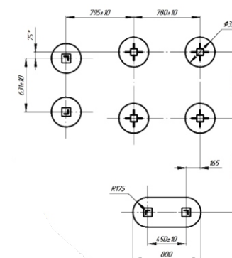
ПЛАН ОБОРУДОВАНИЯ В ОСЯХ
